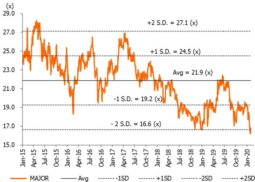
Figure 2: PE Band
